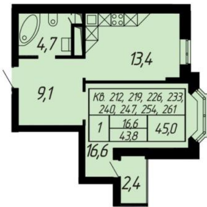
1-комнатная квартира 45,0 кв.м
